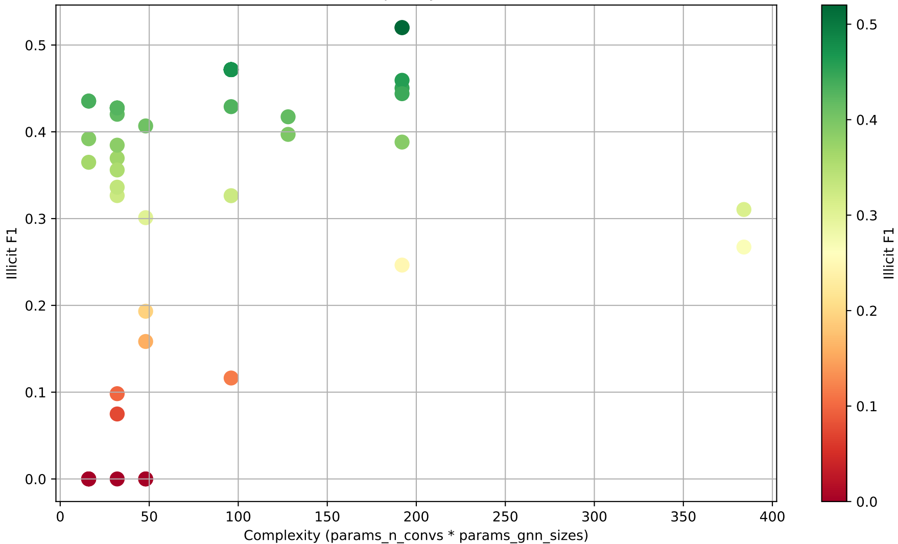
Illicit F1 vs Complexity for AMLSim 1/20
